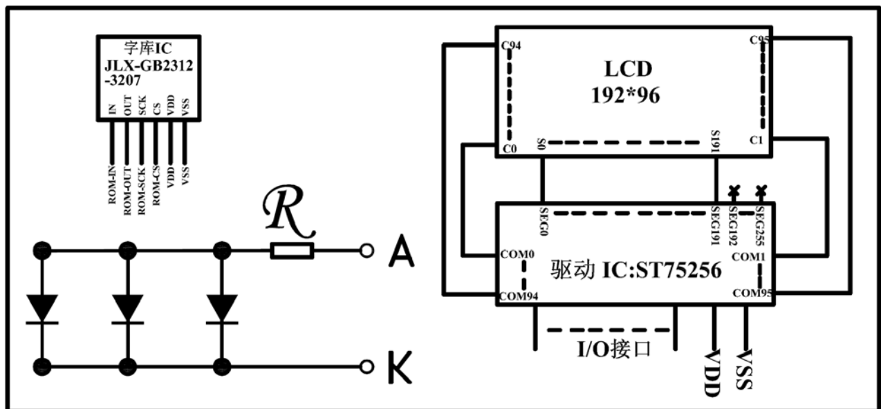
图 2: JLX19296G-91802 电路框图
