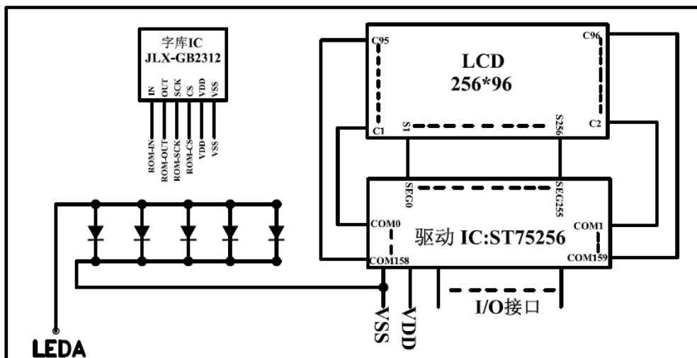
图 2: JLX25696G-968-PL 电路框图
