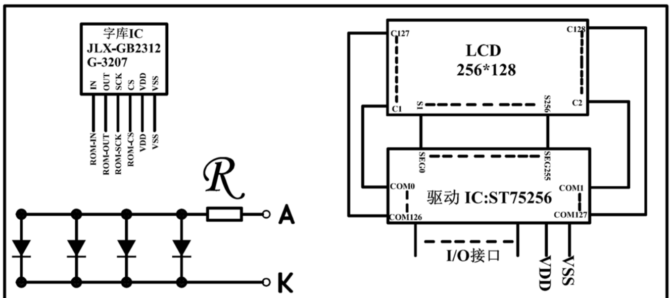
图 2: JLX256128G-920-PL 电路框图
