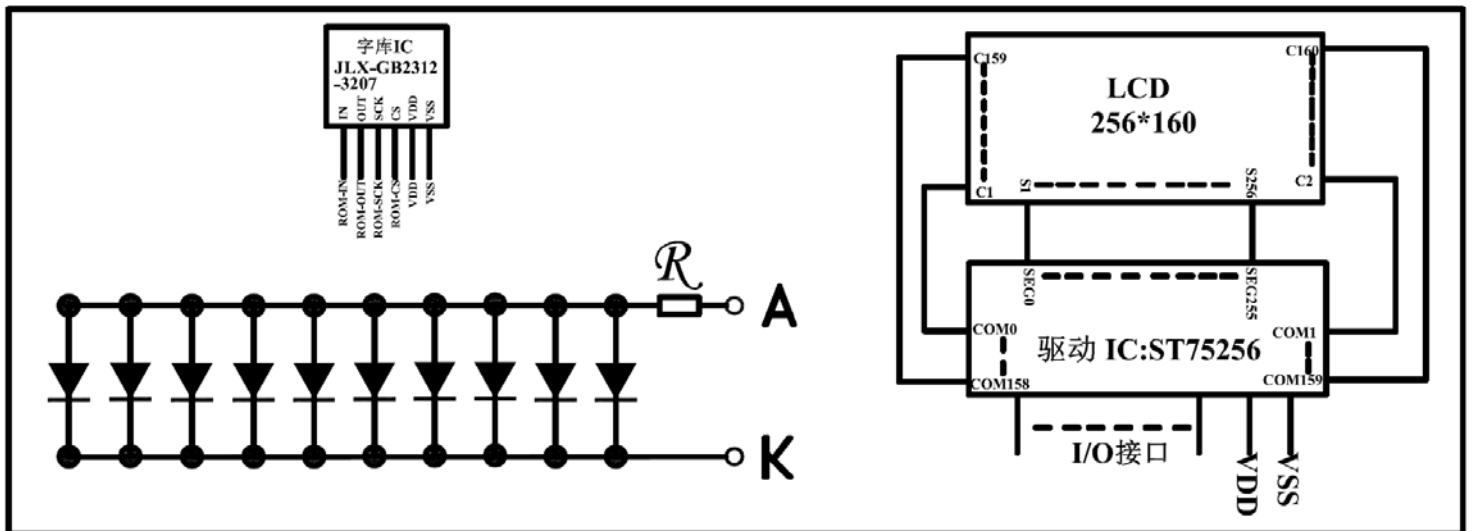
图 2: JLX256160G-922-PL 电路框图
