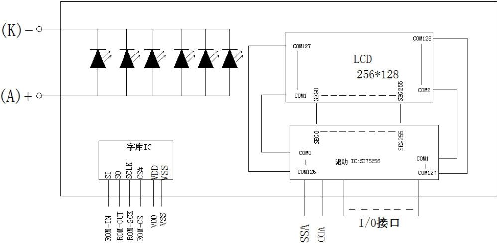
图 2: JLX256128G-929-PL 电路框图
