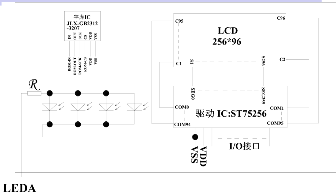
图 2: JLX25696G-967-PL 电路框图
