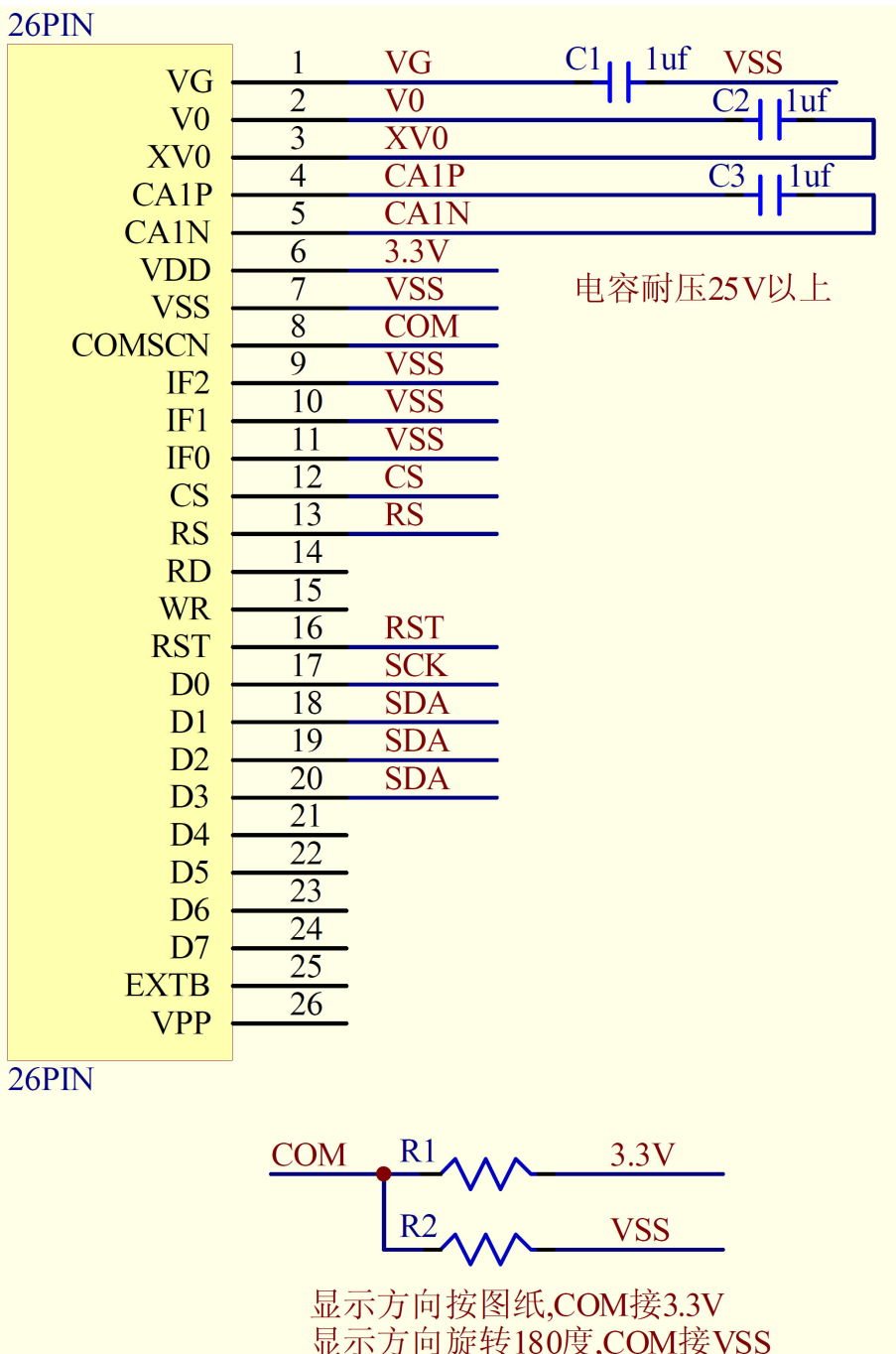
图 9. 串行接口
